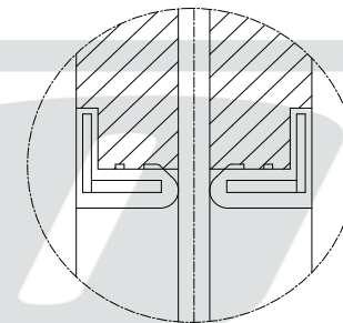
Detail A ® beidseitig weichdichtend
