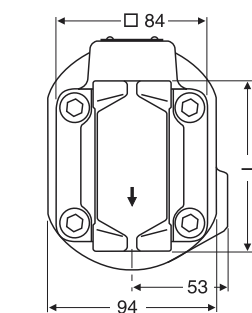
UNA 14Pv mit Gewindemuffen
