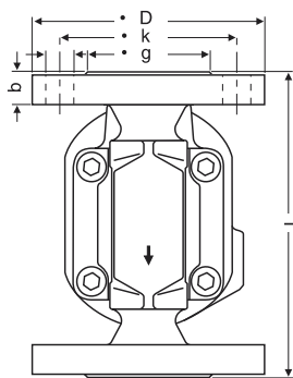
UNA 14v / UNA 16v, mit Flanschen
