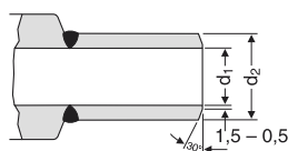
Rohrschweißenden (RSE) (UNA 16)
