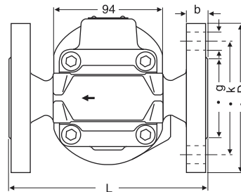
UNA 14h / UNA 16h, mit Flanschen
