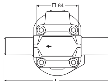
UNA 16h, mit Rohrschweißenden
